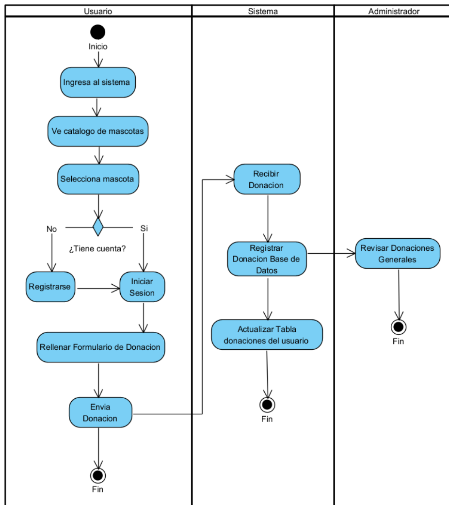
Diagrama de proceso de donación
