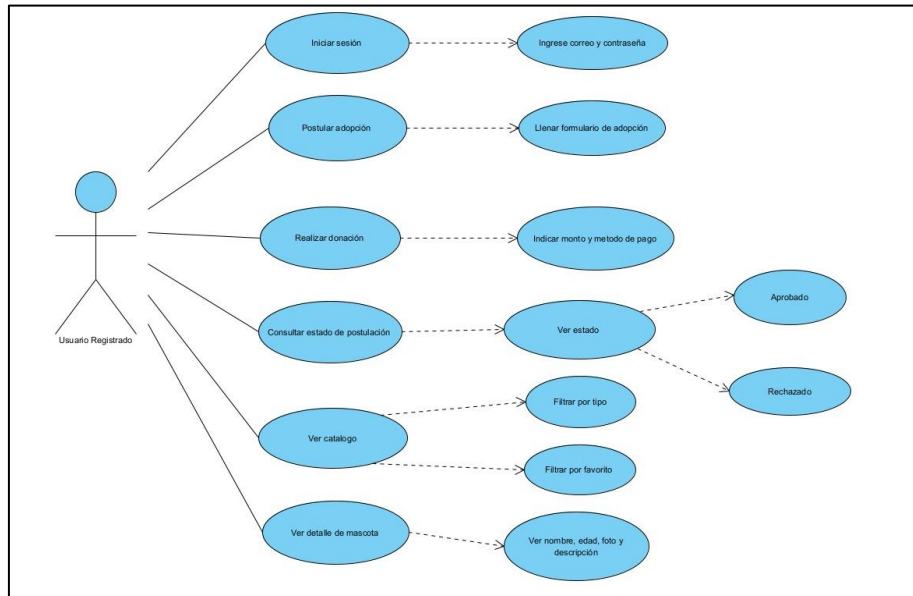
Diagrama de casos de uso para el Usuario
