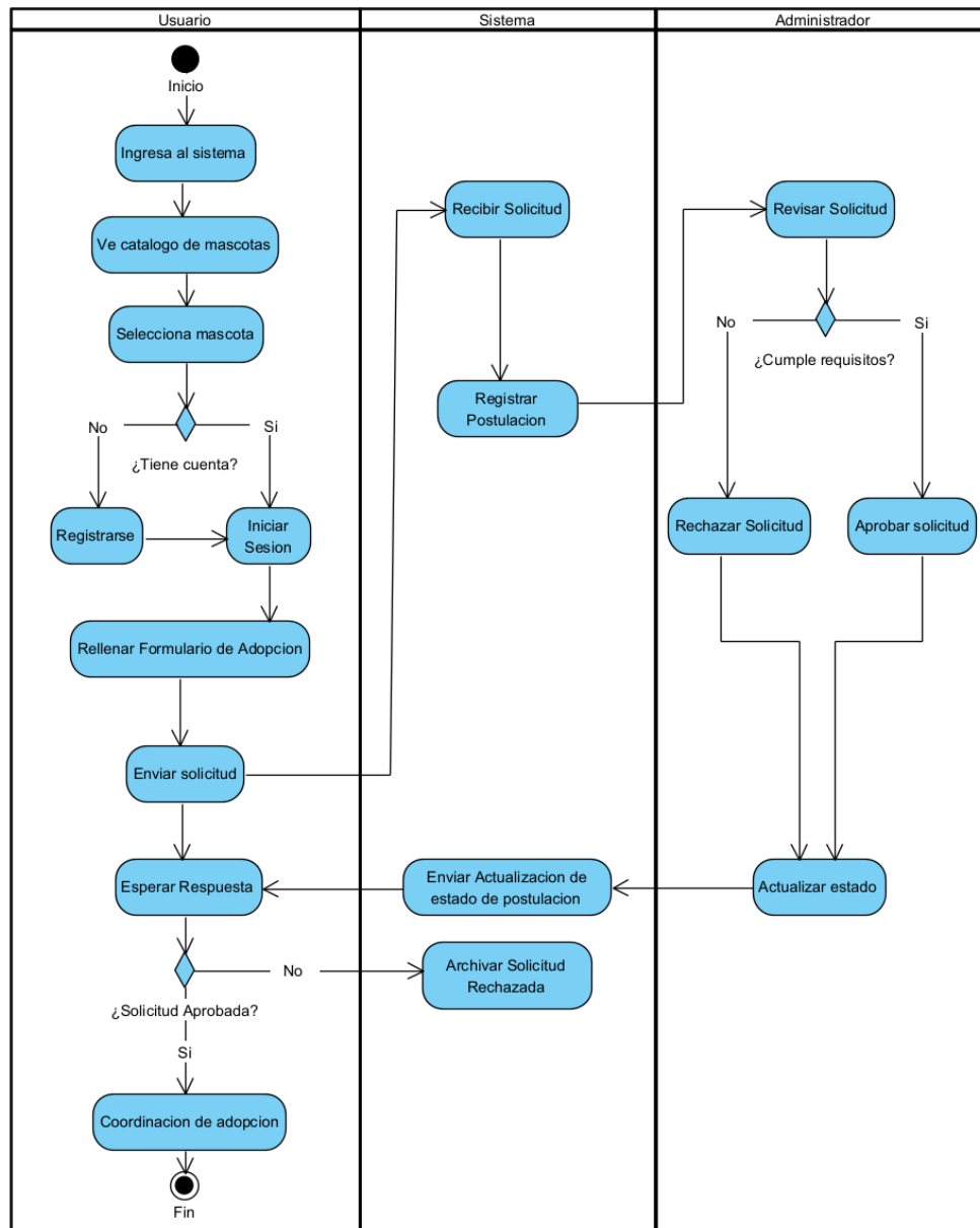
Diagrama de proceso de adopción
